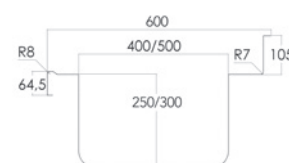
MEDIDAS CUBETA
