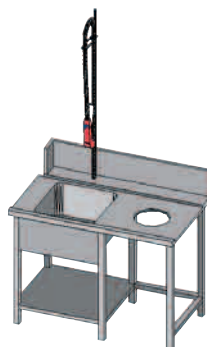
MFDH-1200 LM-D , con fregadero y grifo duchay hueco para cubo
